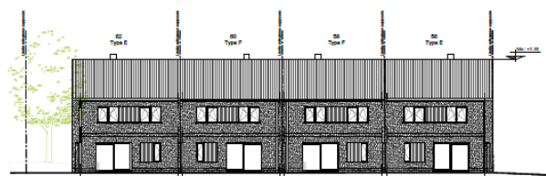
BLOC 1 - Rue Grand'Peine - Elévation Arrière
